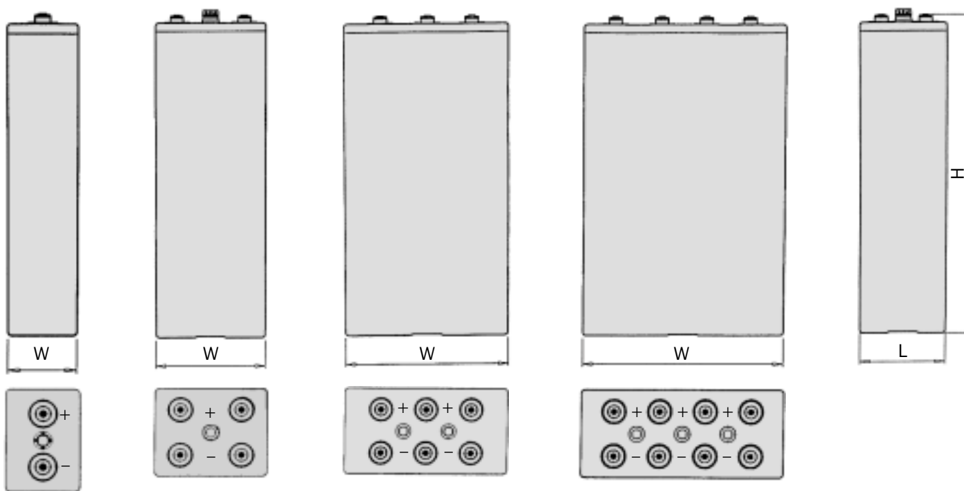
4 OPzS 200 - 6 OPzS 600
